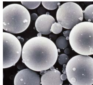
球状溶融シリカの電子顕微鏡写真
