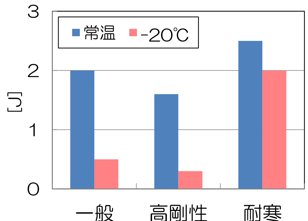
〈デュポン衝撃強度〉 JIS K-7211 準拠
