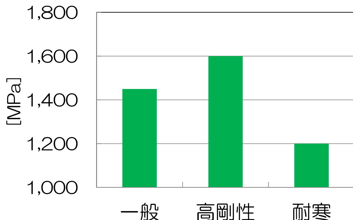
〈引張弾性率〉 JIS K-7113
