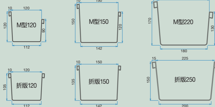
軒どい断面図(単位:mm)
