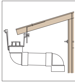
鉄骨スレート（一般地域）
