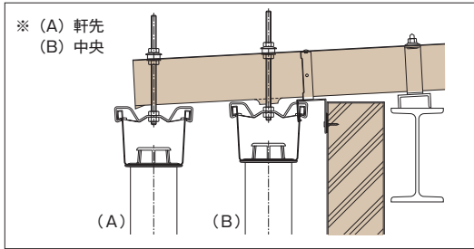
折版屋根（一般地域）
