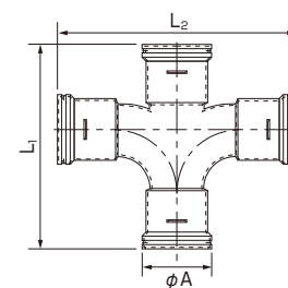
同径 φ50~100
