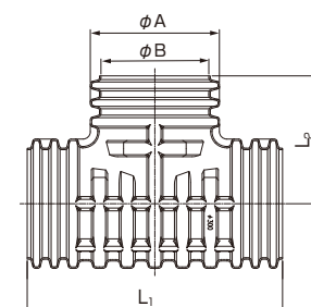
90°チーズ
