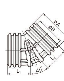
45°エルボ
