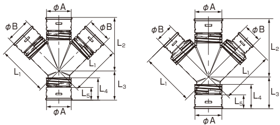
同径 φ150
