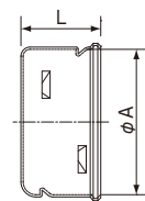
φ50~200
