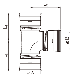
同径 φ100, 150, 200
