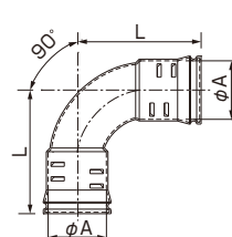
φ50, 80
