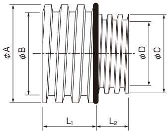
TDW250×200~TDW1000×900
