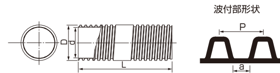
構造図
