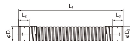
φ150, φ200
