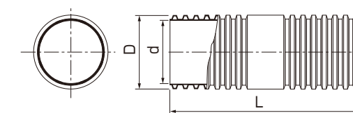
無孔管 H
