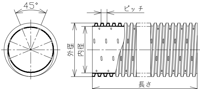
TDW350 2/3Y~500 2/3Y: 千鳥開孔
