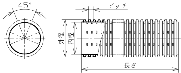
TDW75 2/3Y~200 2/3Y: 每谷開孔
