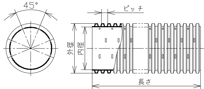
TDW250 2/3Y~300 2/3Y: 千鳥開孔
