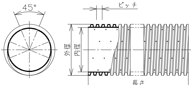
TDW600 2/3Y~1000 2/3Y: 千鳥開孔
