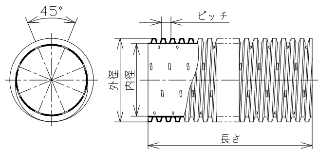
TDW350Y~500Y：千鳥開孔
