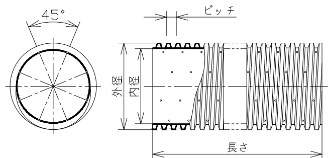
TDW350Y~500Y：千鳥開孔
