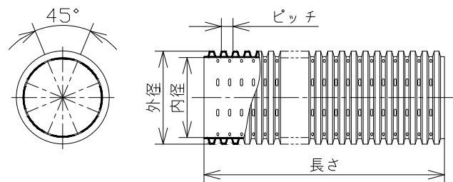
TDW75Y~200Y：毎谷開孔
