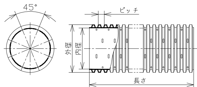
TDW250Y~300Y：千鳥開孔
