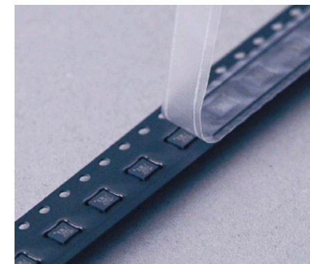
キャリアテープ用シート使用例
