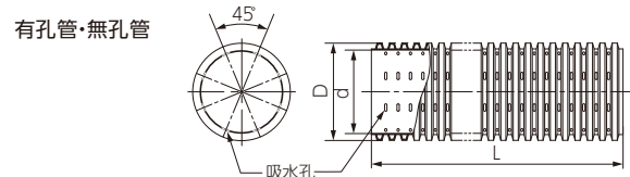
製品構造図
