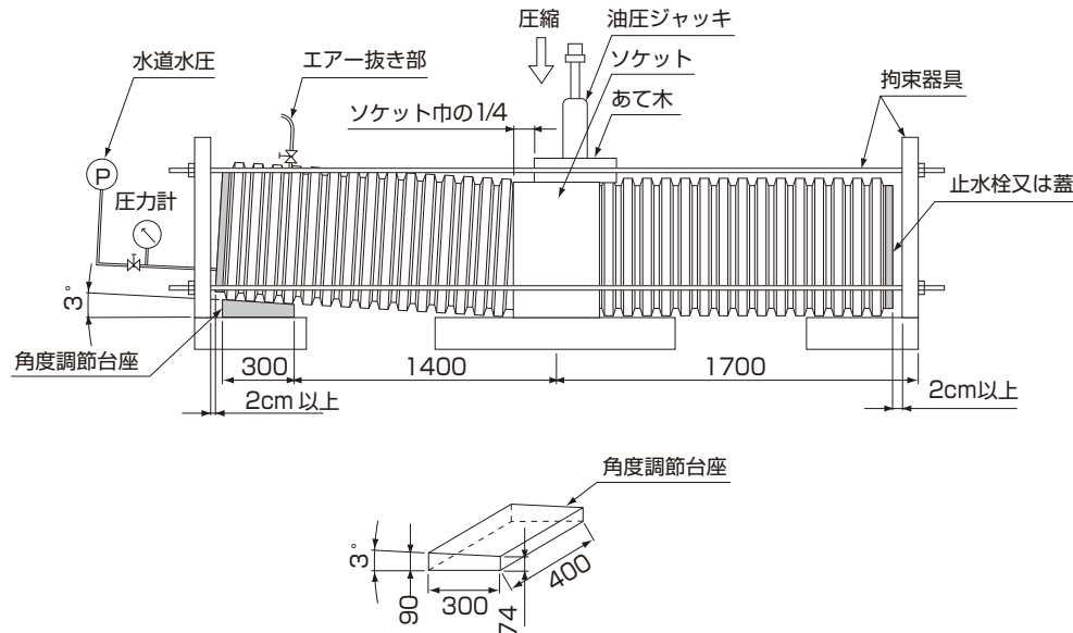
*NEXCO試験方法 126 [=PENK (ポリエチレン波付き管協会)法]
