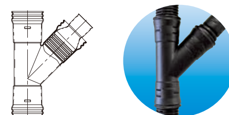
45°チーズφ100 + 片落カラーφ100×75
