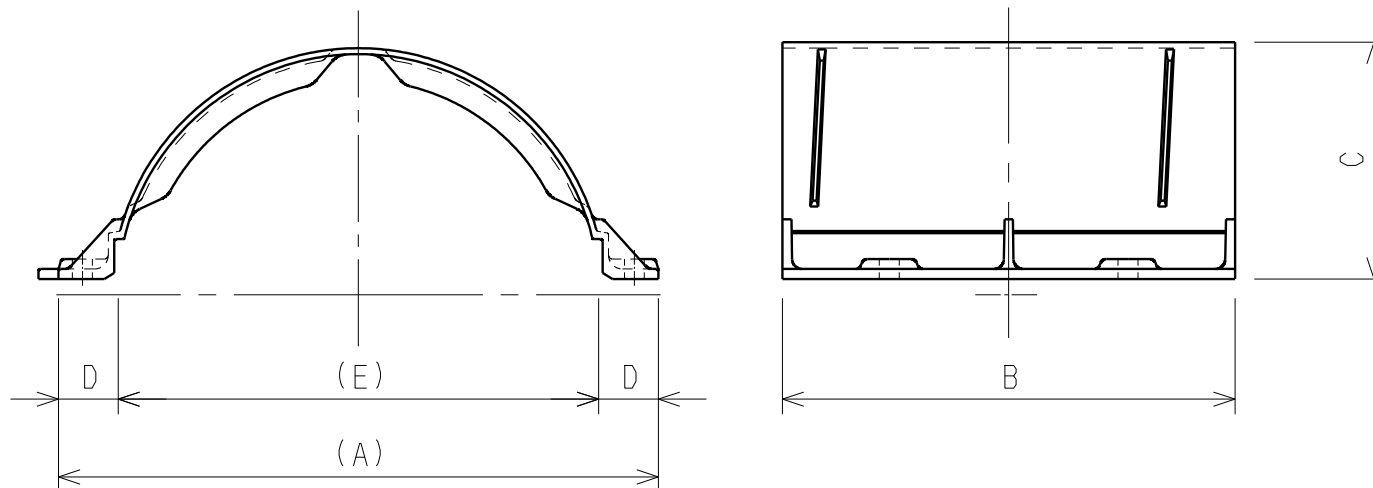
半割型ソケット (2個1組)
