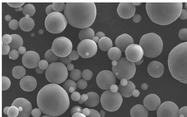
球状氧化铝的电子显微镜照片
